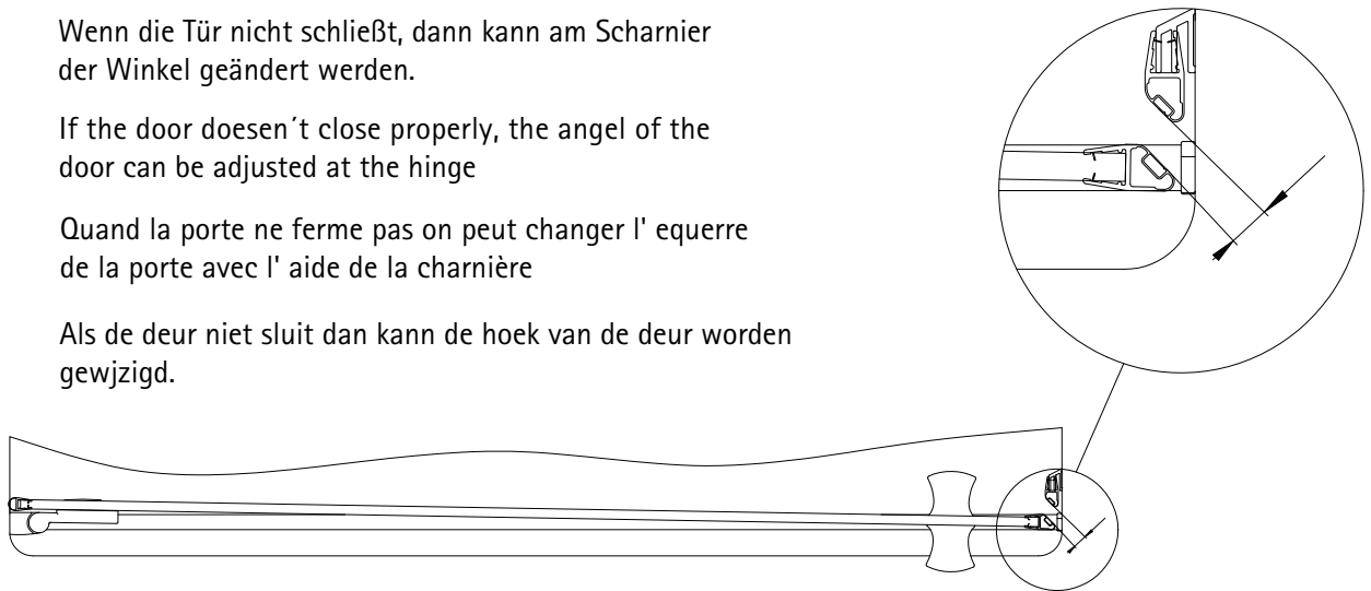
Draufsicht / view from above vue de dessus / bovenaanzicht
